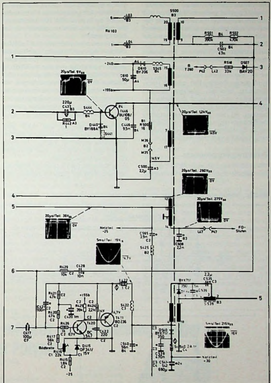
Bild 3b. Teilbild aus der Schaltung der Horizontalendstufe des Philips-Chassis K 9i
