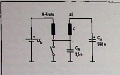
Bild 2. Schaltung zur Erläuterung der Vorgänge nach Bild 1
