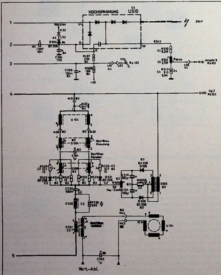
Bild 3c. Teilbild aus der Schaltung der Horizontalendstufe des Philips-Chassis K 91
