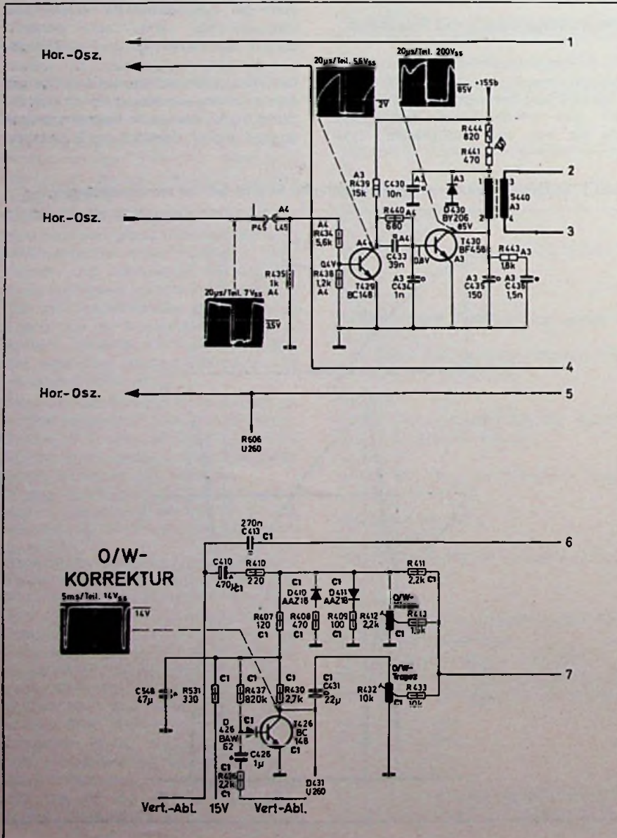
Bild 3a. Teilbild aus der Schaltung der Horizontalendstufe des Philips-Chassis K 91
