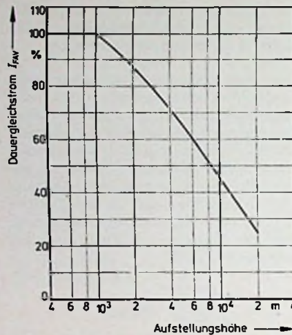
Bild 9. Zulässige Belastbarkeit in Abhängigkeit von der Aufstellhöhe (ITT)
