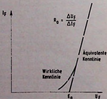
Bild 3. Äquivalente Durchlaßkennlinie (Thomson-CSF)
