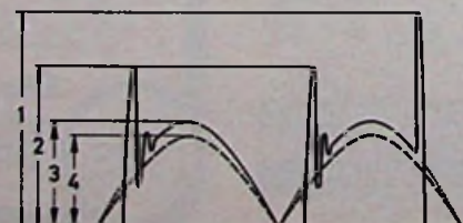
Bild 10. Definition der an einem Gleichrichter auftretenden Sperrspannungen
