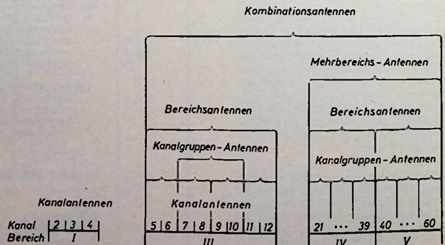
Bild 4.03. Antennenarten mit verschiedenen Frequenzbandbreiten
