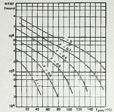
Bild 11. Lebensdauerkurve in Abhängigkeit von der Umgebungstemperatur mit dem Reduktionsfaktor F als Parameter (Thomson-CSF)
