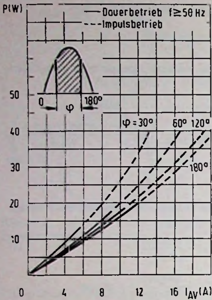
Bild 2. Durchlaßverlustleistung in Abhängigkeit vom mittleren Gleichstrom und dem Stromflußwinkel für Sinushalbwellen (Thomson-CSF)
