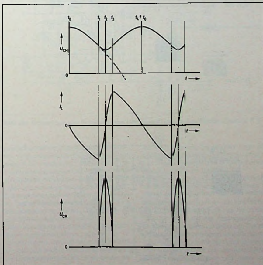
Bild 1. Zeitlicher Verlauf der Spannungen und Ströme bei der Horizontalablenkung
