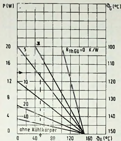
Bild 6. Maximale Verlustleistung in Abhängigkeit von der Umgebungstemperatur und des Wärmewiderstandes des Kühlkörpers (Thomson-CSF)
