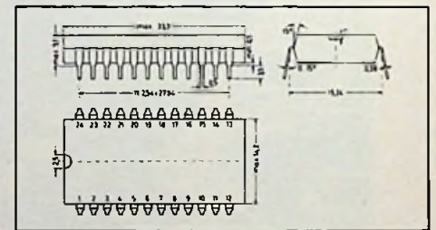
SAA 1050, SAA 1051 im Kunststoffgehäuse 20 B 24 nach DIN 41866 Gewicht ca. 3,5 g Maße in mm
