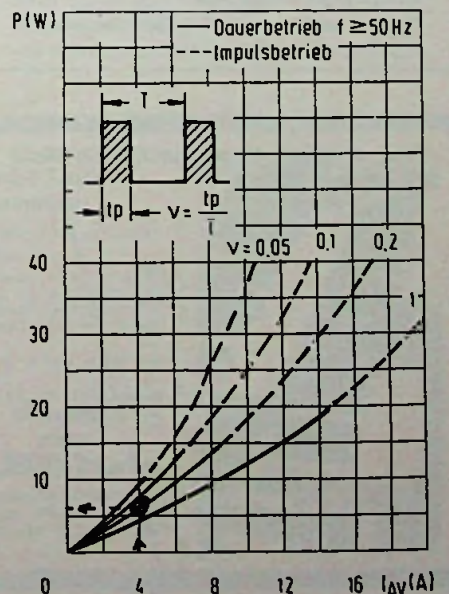
Bild 1. Durchlaßverlustleistung in Abhängigkeit vom mittleren Gleichstrom und dem Tastverhältnis für Rechteckimpulse (Thomson-CSF)
