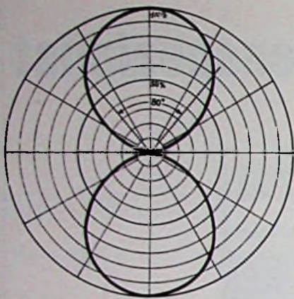
Bild 4.01. Normierte Horizontal-Richtkennlinie des Halbwelldipols
