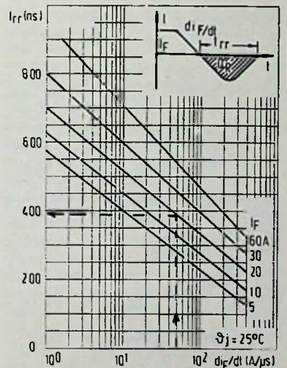
Bild 7. Sperrverzögerungszeit t_{rr} in Abhängigkeit vom Durchlaßstrom I_F . I_R wird durch den Lastkreis nicht begrenzt (Thomson-CSF)
