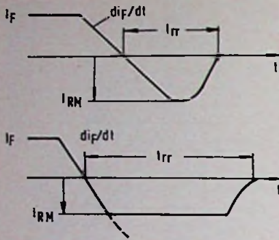
Bild 8. Darstellung zur Berechnung der Sperrverzögerungszeit (Thomson-CSF)
