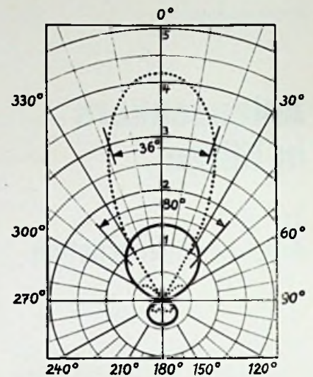
Bild 4.02. Horizontalrichtkennlinien ----- 2-Element-Antenne mit Anschlußdipol und Reflektor ..... 20-Element-Antenne mit Anschlußdipol, drei Reflektoren und sechzehn Direktoren
